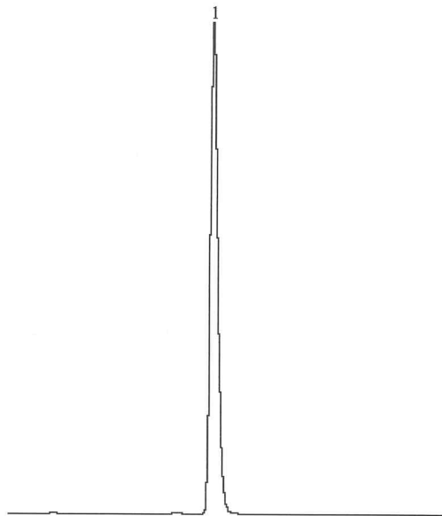
图 1 灭草松水剂的高效液相色谱图
